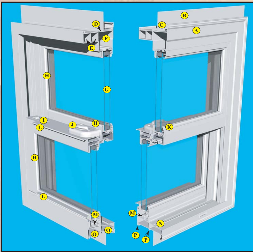
Optional Cam Lock
